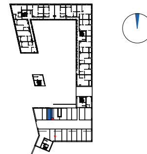
VENDNDODHJA E GARAZHIT NE PLANIN E KATIT NENTOKE SH 1: 2000
